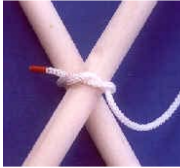
ÇAPRAZ BAĞLAMA
